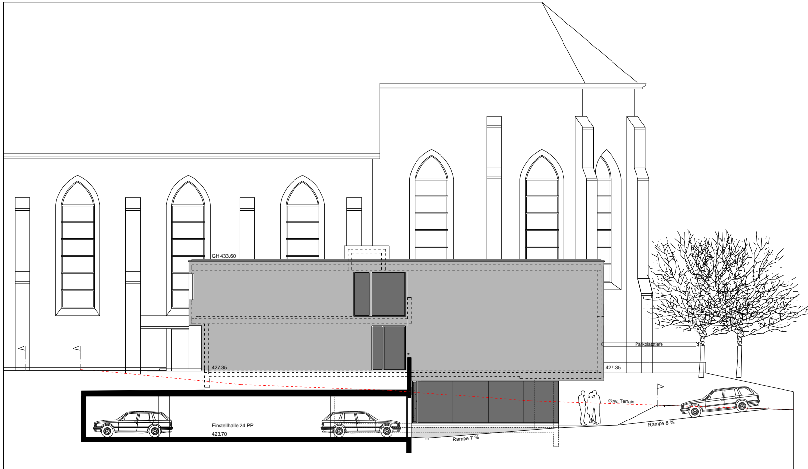
OSTFASSADE
